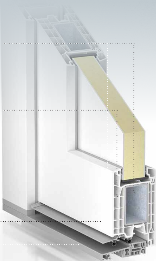
Falzfüllung
